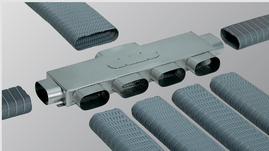
Skrzynka rozdzielcza powietrza System 100/System 150 Rozdzielacz główny, powietrza doprowadzanego i zużytego
