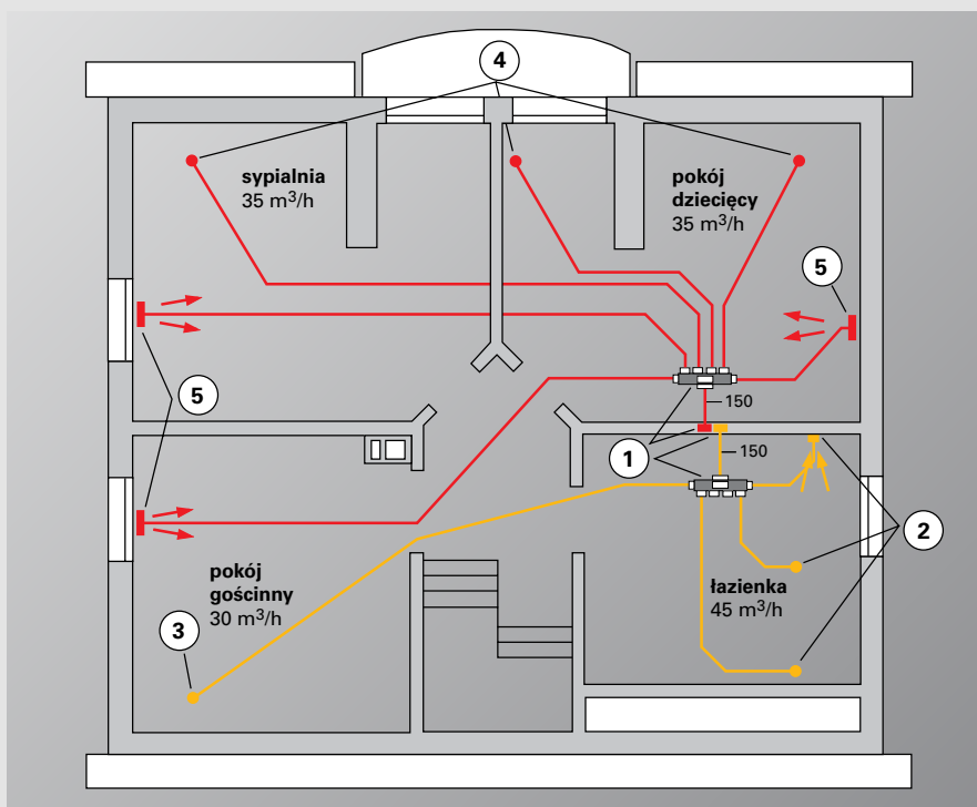
Rzut poziomy rozdziału powietrza na surowej podłodze piętra
