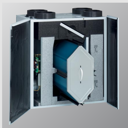
Krzyżowy przeciwprądowy wymiennik ciepła z odzyskiem ciepła ponad 90%
