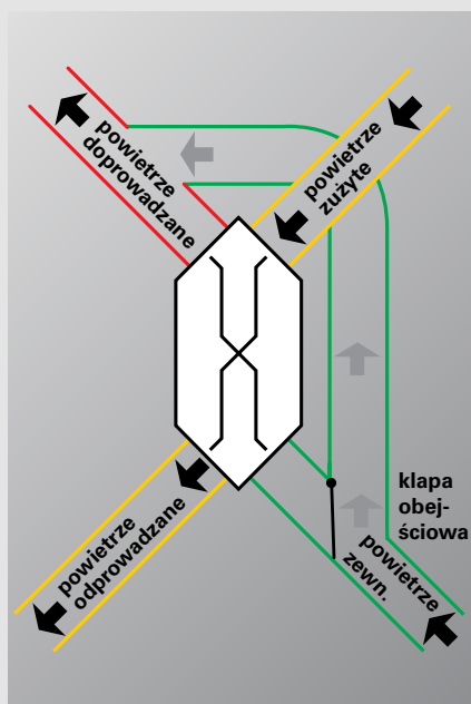
Sposób funkcjonowania zintegrowanej klapy obejścia
