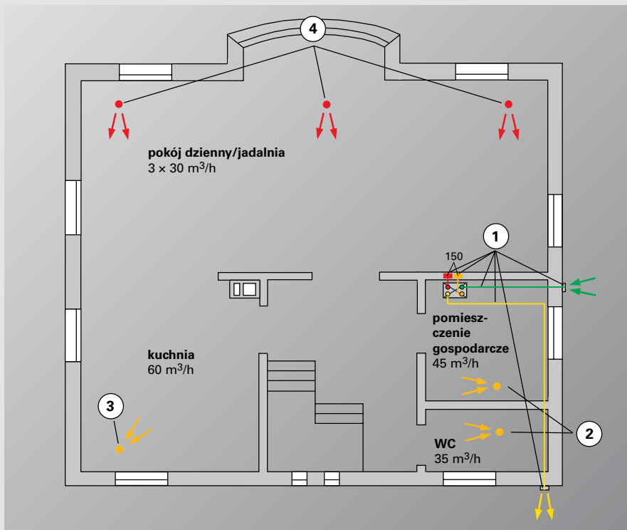
Rzut poziomy parteru – rozmieszczenie zaworów powietrza doprowadzanego i zużytego przez przejścia w suficie, montaż urządzenia w pomieszczeniu gospodarczym
