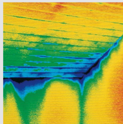
Przebieg temperatury w tym samym narożniku – tutaj może dochodzić do wykrapiania się kondensatu
