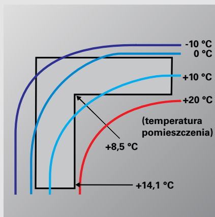
Przebieg temperatury na ścianie zewnętrznej – chłodny narożnik sprzyja powstawaniu grzyba
