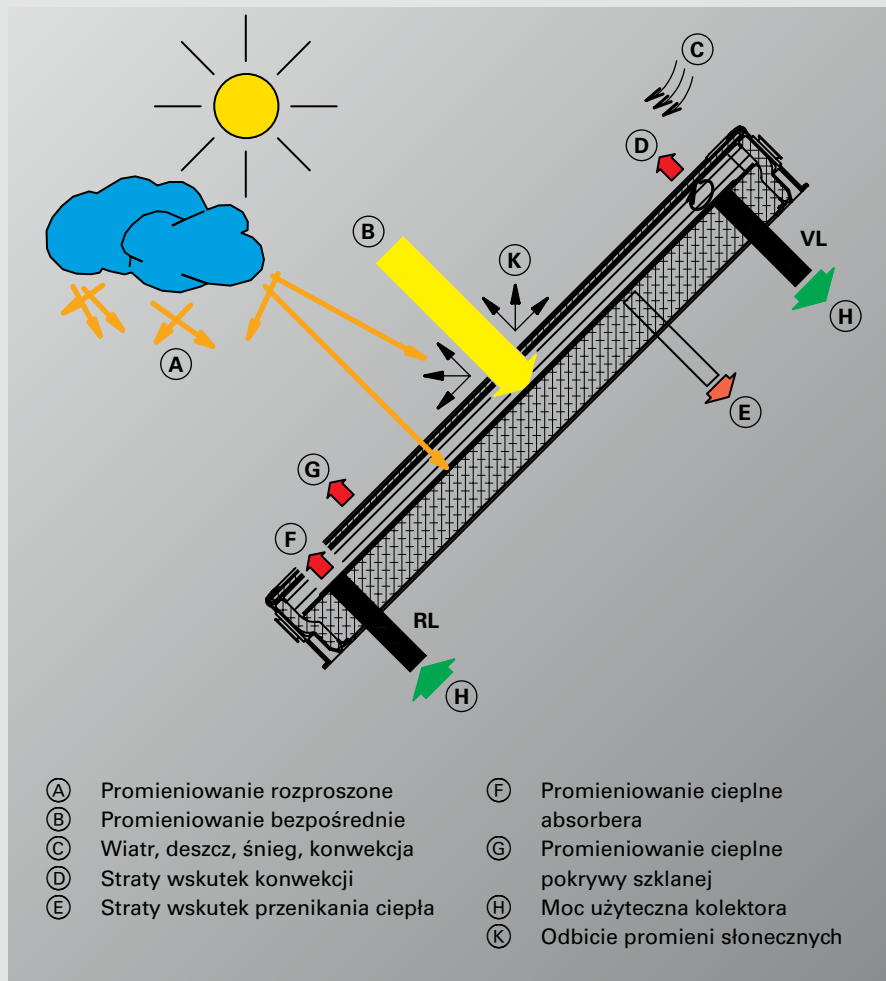
Rys. 2: Wykorzystanie promieniowania słonecznego w kolektorze
