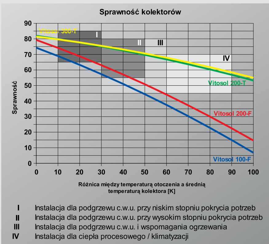
Rys. 10: Sprawności kolektorów
